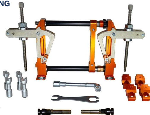
Art. 519 1584 PMM EM RINGSTYR Til delte EM fælge.
